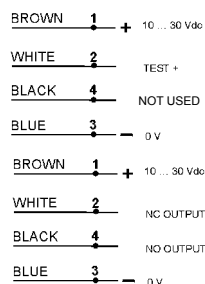
S50-ML/MH-2
