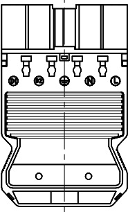
Teil 2: Stecker 640394
