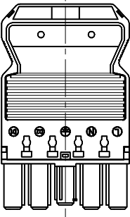
Teil 1: Buchse 640393
