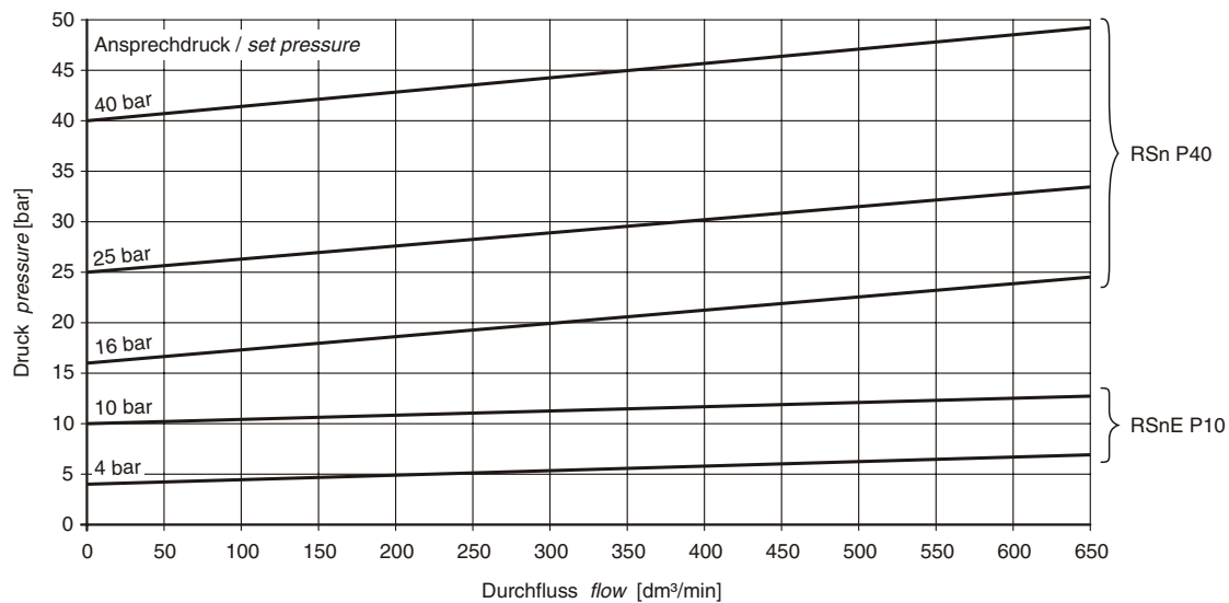
Fig. 7: RSn(E)2
