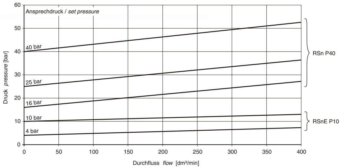
Abb. 6: RSn(E)1.1/2
