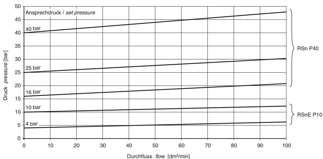
Abb. 4: RSn(E)3/4
