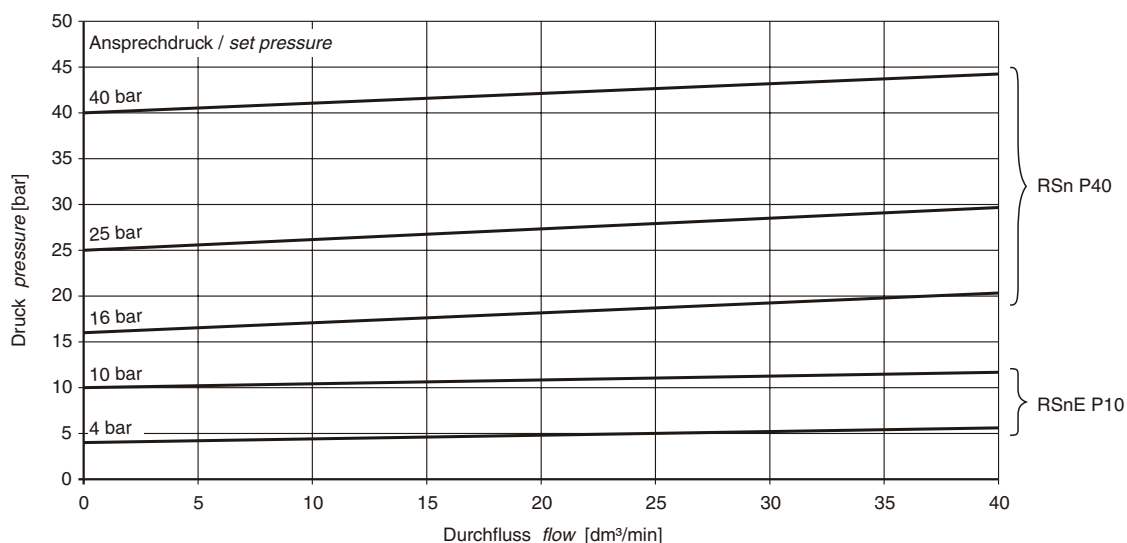
Abb. 3: RSn(E)1/2
