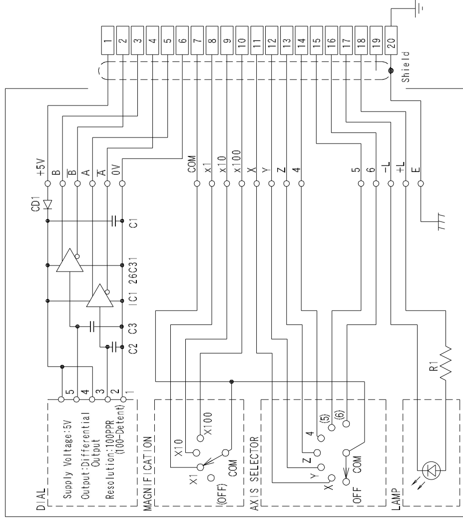
Curl Code Wiring
