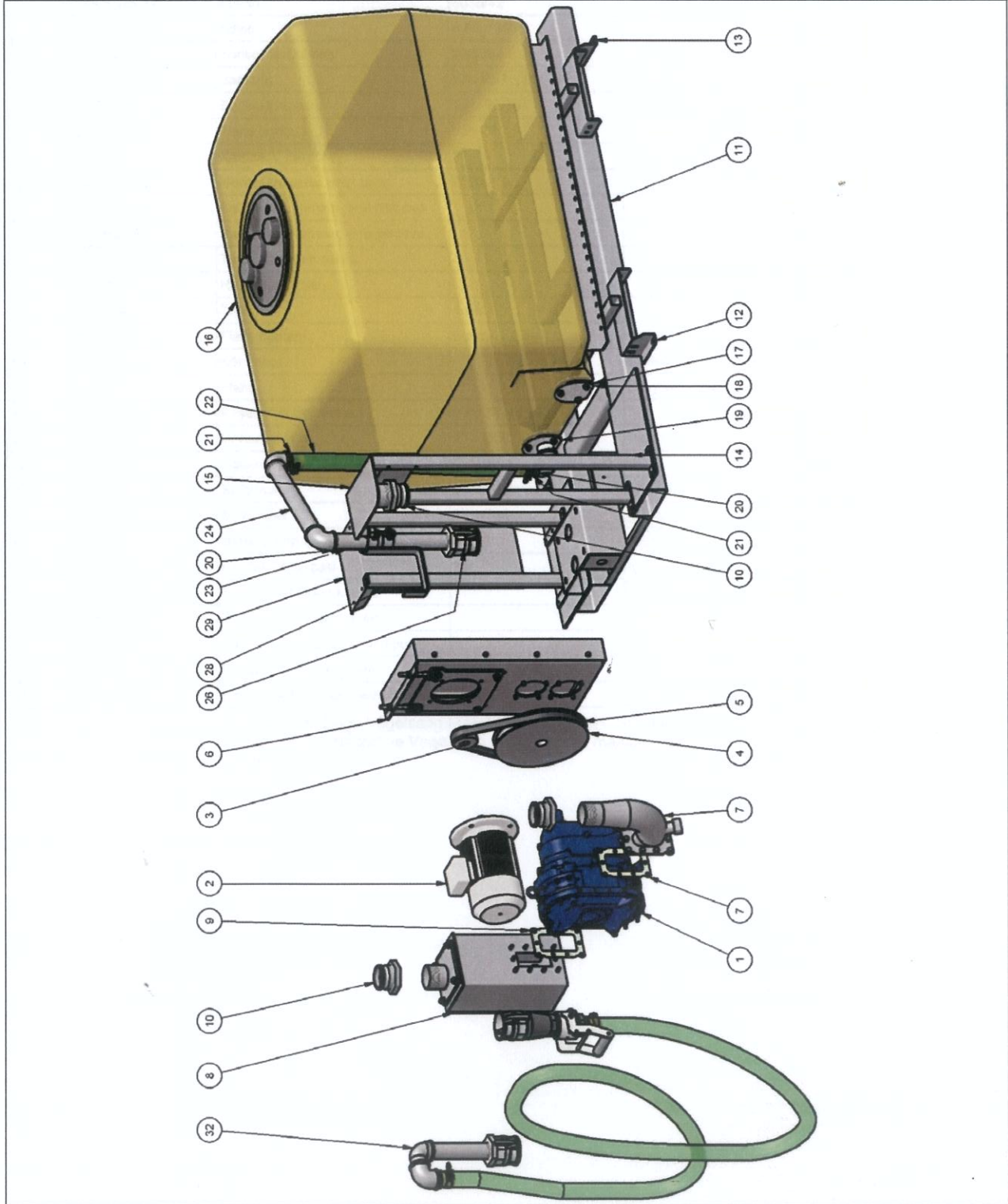
Şekil 2: Yedek/aşınabilir parça listesi - Mobil emme sistemi
