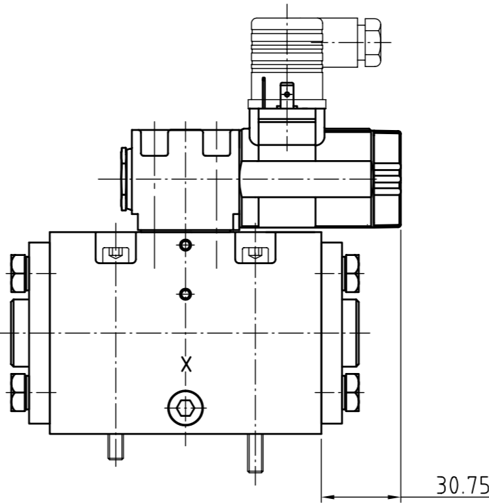
4/2-Wegeventil (M1:2)
