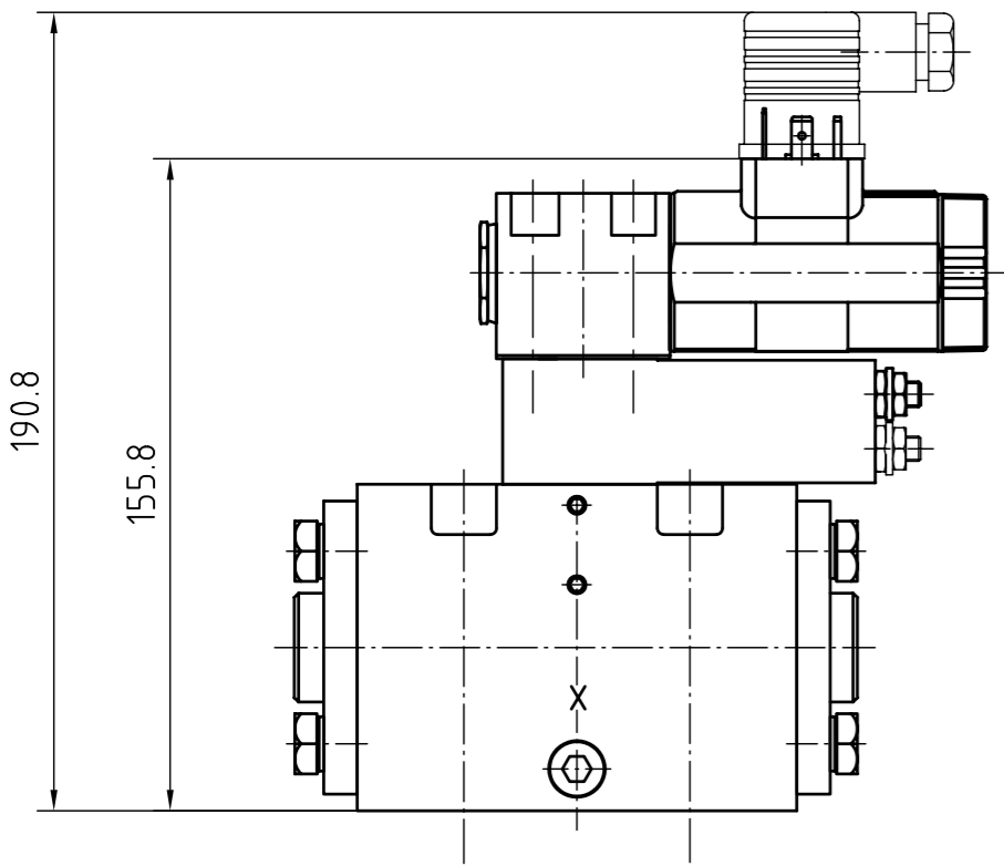
Anschlußbild
