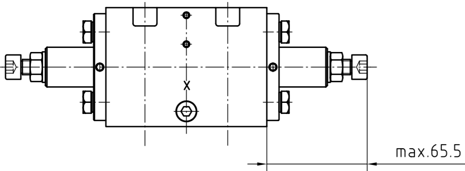
Hubbegrenzung B4 (M1:2.5)
