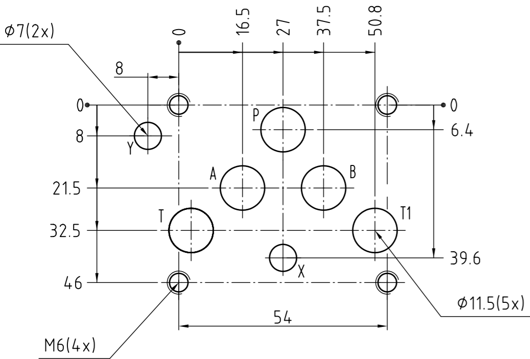
Anschlußbild
