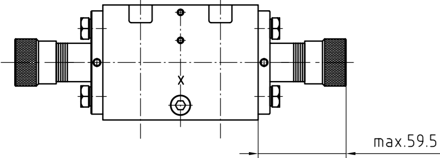
Hubbegrenzung B4 (M1:2.5)
