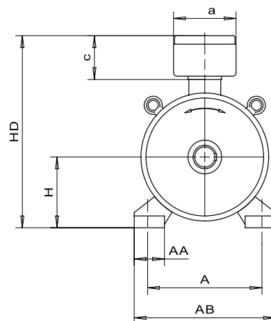
Prinzipskizze Anschlussraum Schematic Diagram Terminal Box
