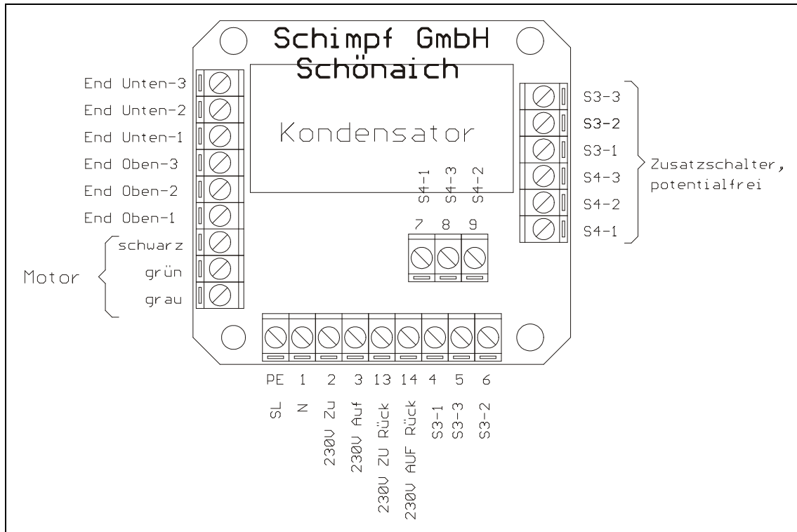
Abbildung 1: AB336 mit 2 Zusatzschalter
