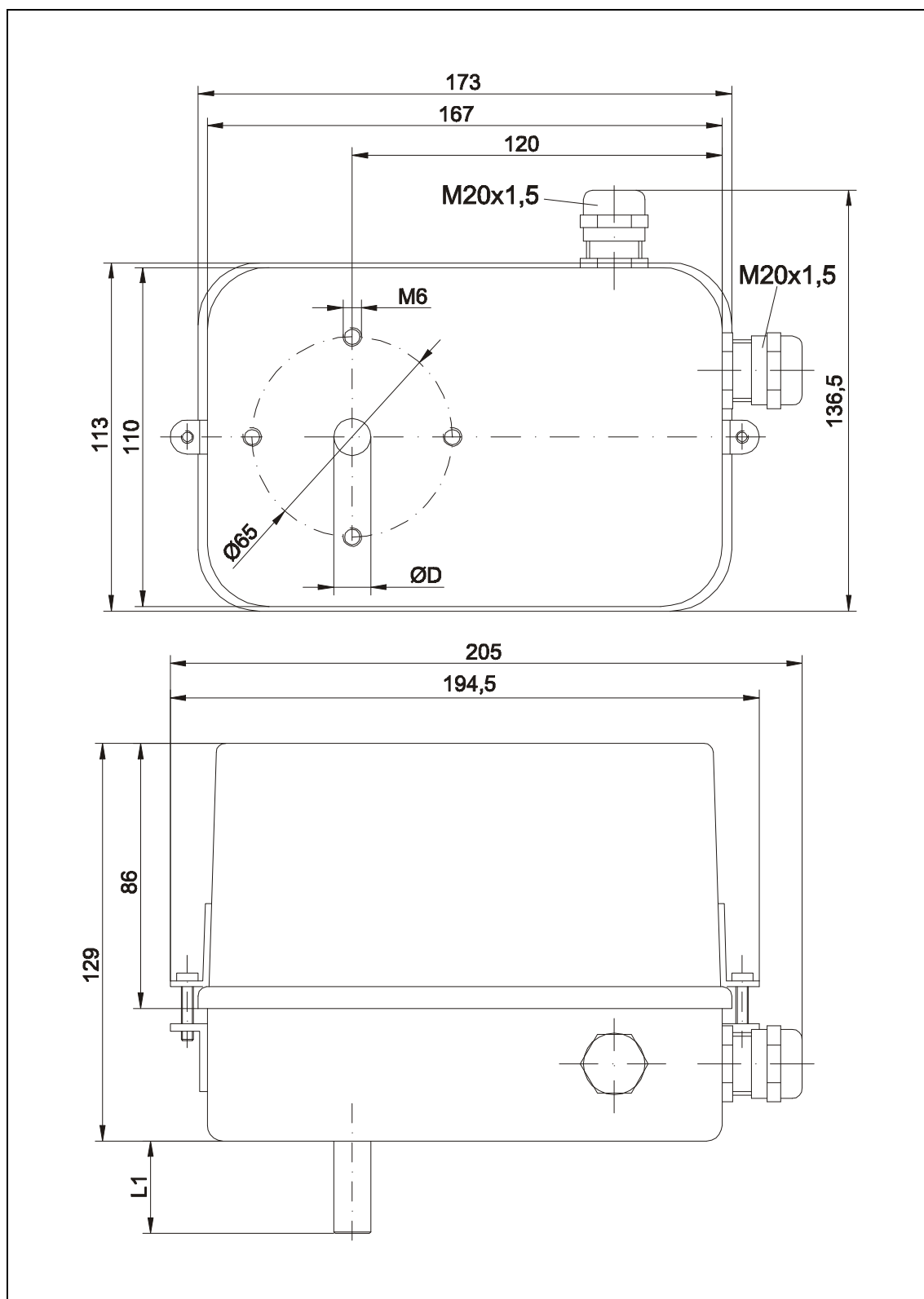
Abbildung 4: Abmessungen Antrieb Typ SM 60 Serie 02
