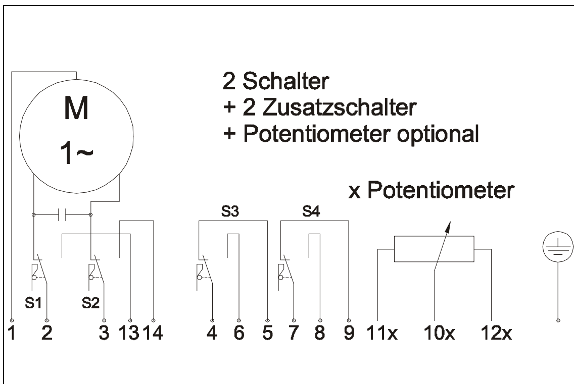
Abbildung 2: AB336 mit 2 Zusatzschalter und 1 Potentiometer
