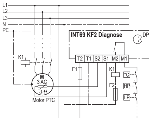
Anschluss-Schaltbild
