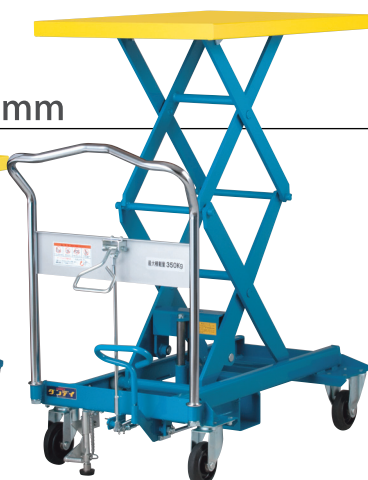
350kg リフト台車 (W シザー) UDA-350W UDA-350WJ (ジャバラ付) 最大積載量 /350kg テーブル寸法 /600×910mm テーブル高さ /345~1265mm
