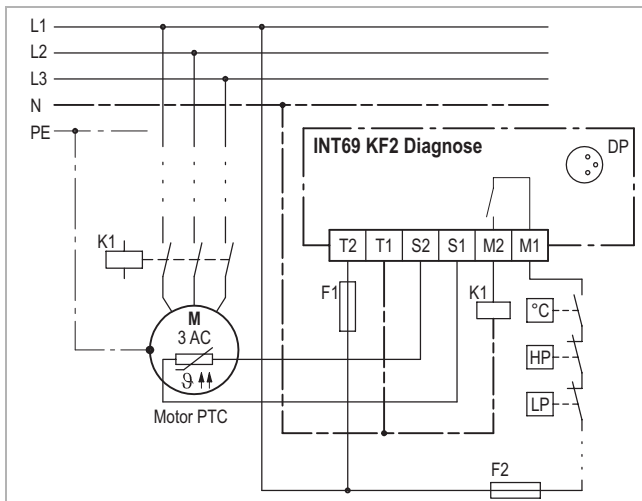
Anschluss-Schaltbild
