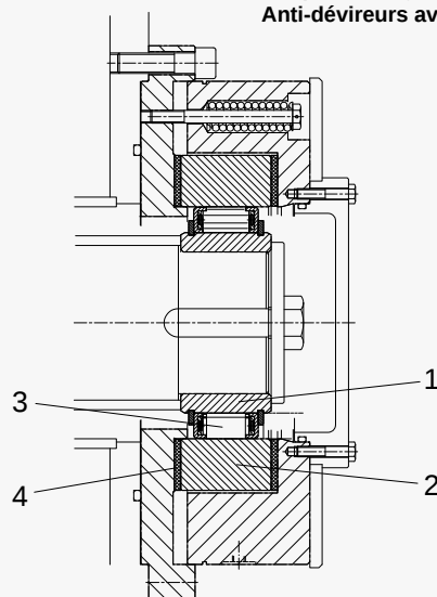
Rücklaufsperren mit Drehmomentbegrenzung 2) Torque limiting backstops Anti-dévireurs avec limitation du couple
