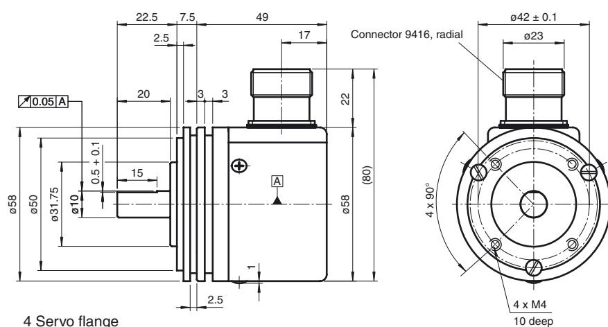
4 Servo flange
