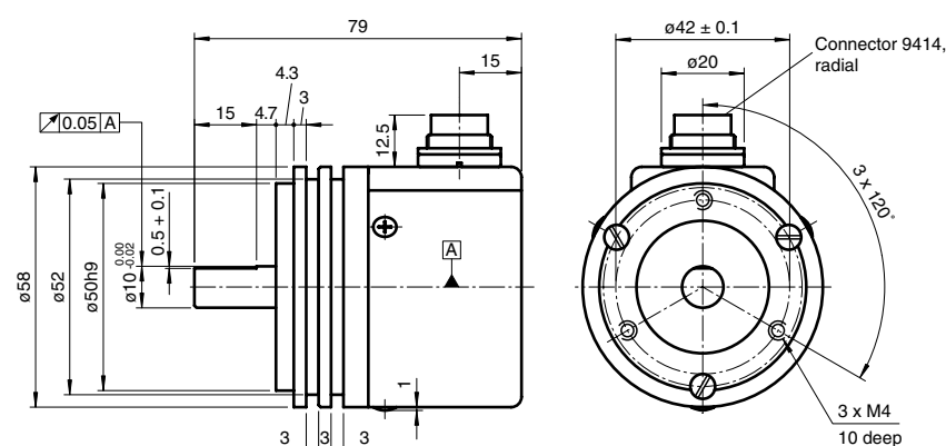
3 Servo flange
