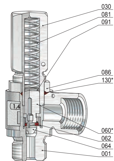
Kopf C Kegel mit O-Ring > 2 [bar(g)]
