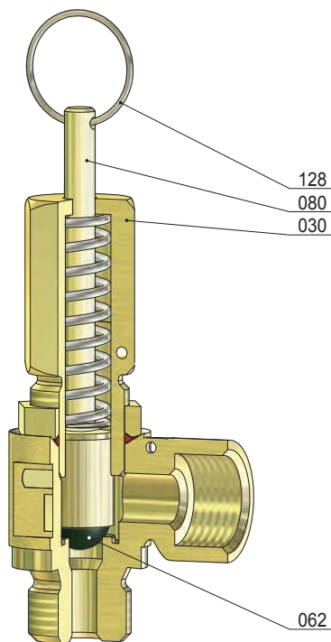
Kopf D nur in Typ 5.3 Kegel mit Kugel < 2 [bar(g)]
