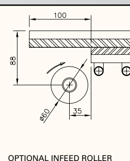
OPTIONAL INFEED ROLLER
